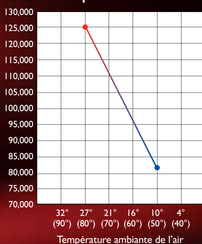
Capacité de chauffage en BTU/heure UltraTemp 120 et 120 R H/C
