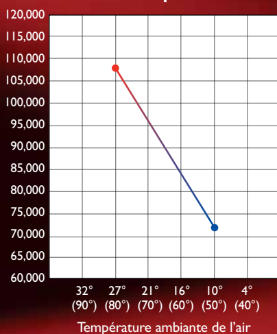
Capacité de chauffage en BTU/heure UltraTemp 110
